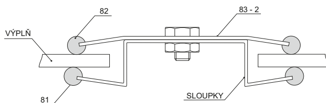
Střešní sloupky
